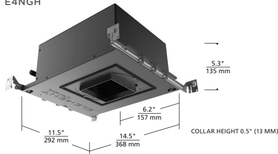
IC AIRTIGHT / NON-IC AIRTIGHT / CHICAGO PLENUM (29W)
