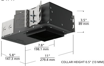
IC AIRTIGHT / NON-IC AIRTIGHT / CHICAGO PLENUM (UP TO 24W)
