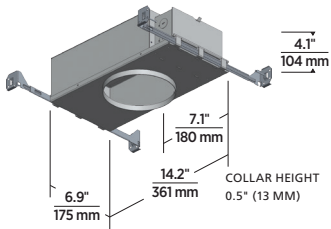
5" APERTURE IC AIRTIGHT / CHICAGO PLENUM
