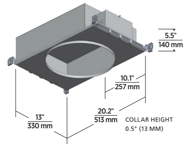
12" APERTURE IC AIRTIGHT / CHICAGO PLENUM
