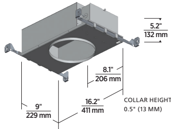
8" APERTURE IC AIRTIGHT / CHICAGO PLENUM
